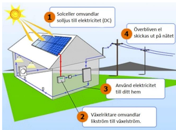
Bilden visar typfunktion av solceller
